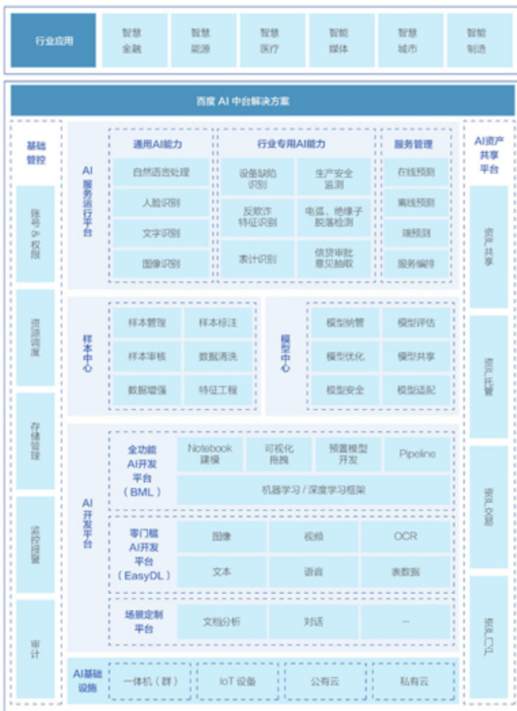
图 百度 AI 中台体系架构
