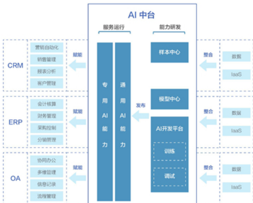
图 AI中台打破传统烟囱式业务壁垒
