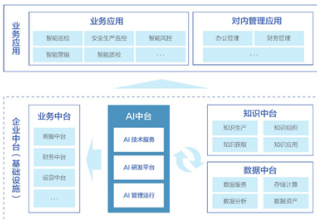
图 AI 中台的定位
